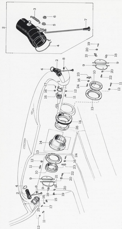
FIG.-107 VENTILATOR AIR DUCT
